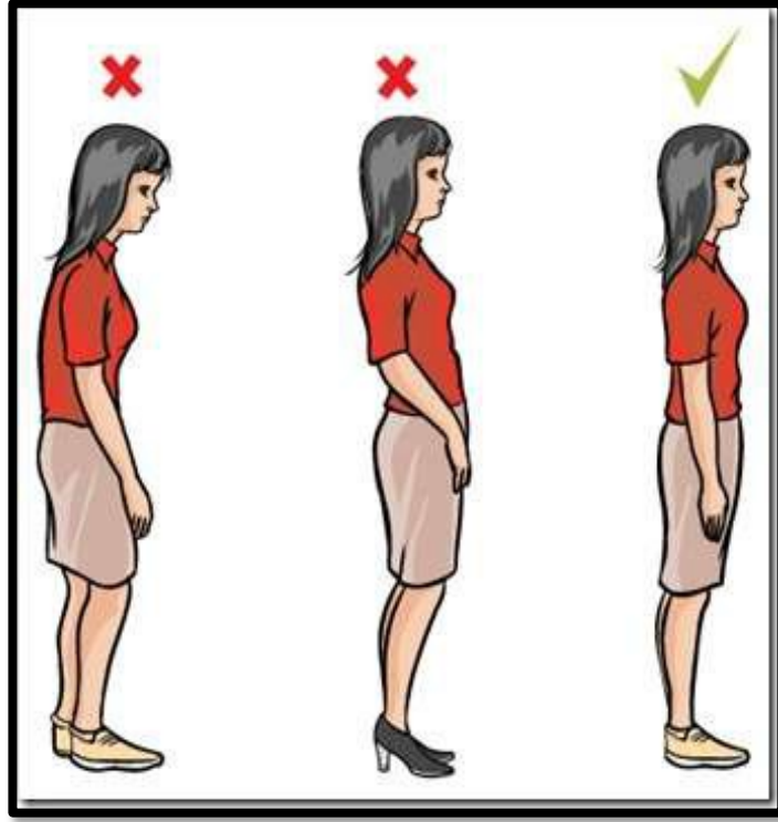
Şekil 12.1. Beden Duruşu
