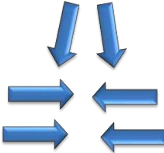
Şekil 12.5. Ayakların Konumu
