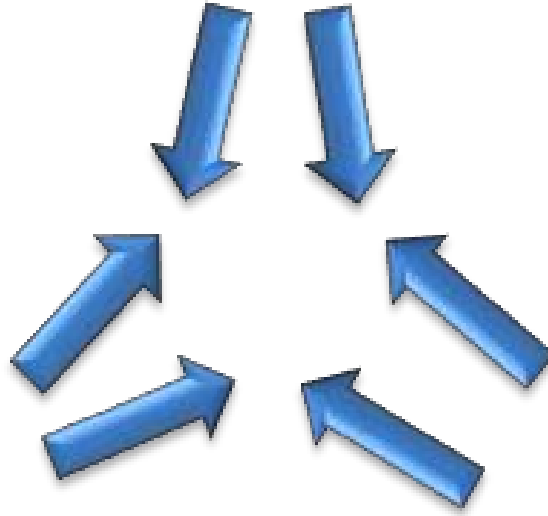
Şekil 12.4. Ayakların Konumu
